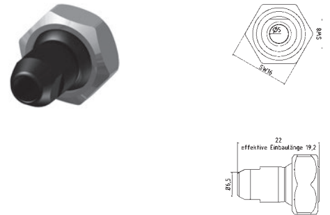
KU-1-DU-50 Kunststoff-Düse gerade Bohrung Ø 5,0 mm plastic nozzle straight Ø 5,0 mm
