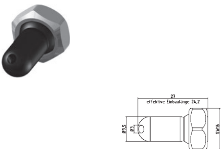
KU-1-DU-60 Kunststoff-Düse 60° Bohrung Ø 3 mm plastic nozzle 60° drill hole Ø 3 mm
