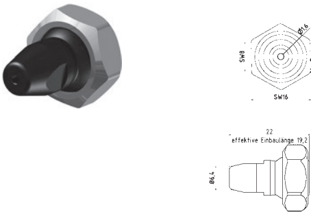
KU-1-DU-16 Kunststoff-Düse gerade Bohrung Ø 1,6 mm plastic nozzle straight Ø 1,6 mm
