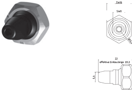
KU-1-DU-32 Kunststoff-Düse gerade Bohrung Ø 3,2 mm plastic nozzle straight Ø 3,2 mm
