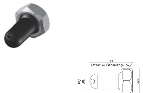
KU-1-DU-30 Kunststoff-Düse 30° Bohrung Ø 3 mm plastic nozzle 30° drill hole Ø 3 mm
