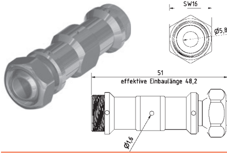
1-DU-EL3 Duschelement mit Bohrungen 3 x Ø 1,6 mm shower element drillings 3 x Ø 1,6 mm
