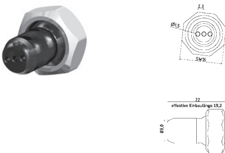
KU-1-DU-3-16 Kunststoff-Düse gerade Bohrung 3 x Ø 1,6 mm plastic nozzle straight 3 x Ø 1,6 mm
